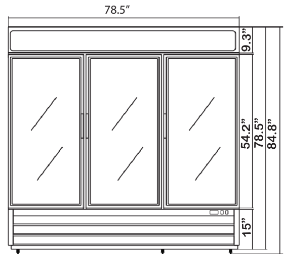
SG1.9L3-HC Swing Door
